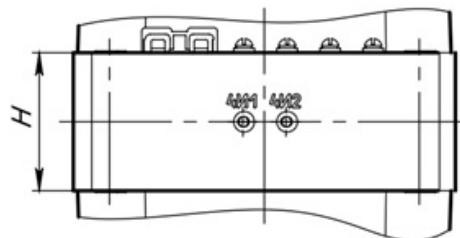
Рис. А.4 – Панель контактов трансформатора тока ТПОЛ-СВЭЛ-10-4 Остальное см. рис. А.1.
