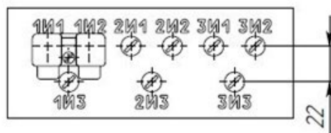
Рис. А.10 – Панель контактов трансформаторов тока ТПОЛ-СВЭЛ-10-3.1 Остальное см. рис. А.7
