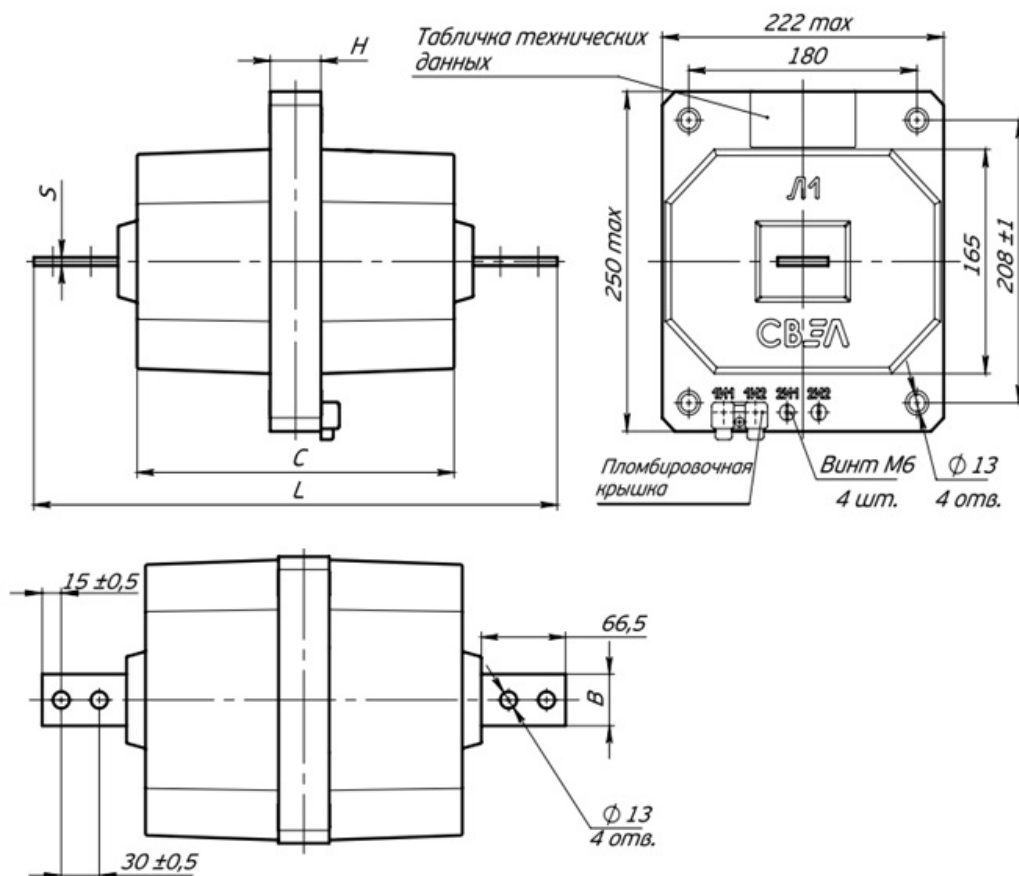
Рис. А.1 – Общий вид трансформатора тока ТПОЛ-СВЭЛ-10-2 на номинальные первичные токи 5-200 А и ТПОЛ-СВЭЛ-10-3 на номинальные первичные токи 5-400 А.
