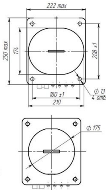
Рис. А.8 – Общий вид трансформатора тока ТПОЛ-СВЭЛ-10-2.1(3.1) на номинальные первичные токи 500-1000 А Остальное см. рис. А.7
