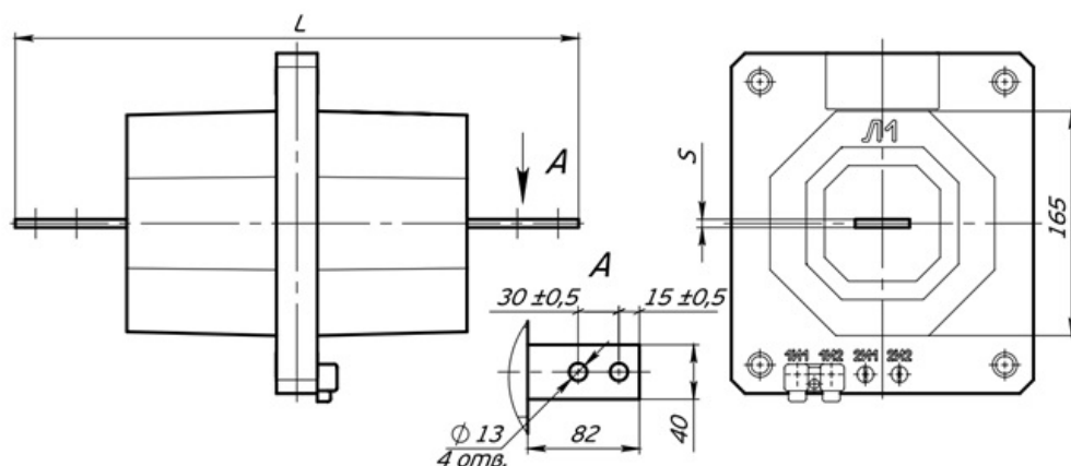
Рис. А.2 – Общий вид трансформатора тока ТПОЛ-СВЭЛ-10-2 на номинальные первичные токи 300-1000 А и ТПОЛ-СВЭЛ-10-3 на номинальные первичные токи 600-1000 А. Остальное см. рис. А.1.
