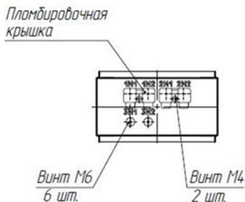
Рис. А.13 – Панель контактов трансформатора тока ТПОЛ-СВЭЛ-10М-3. Остальное см. рис. А.11
