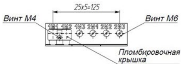
Рис. А.9 – Панель контактов трансформаторов тока ТПОЛ-СВЭЛ-10-2.1 Остальное см. рис. А.7
