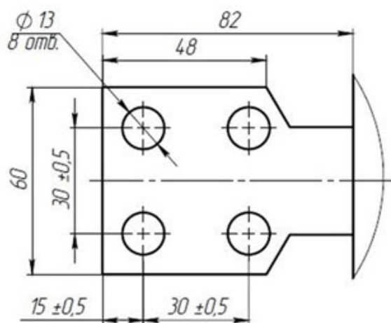
Рис. А.15 – Общий вид трансформатора тока ТПОЛ-СВЭЛ-10М на номинальные первичные токи 1200-2000 А. Остальное см. рис. А.11
