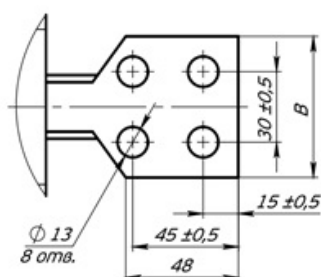
Рис. А.5 – Общий вид трансформатора тока ТПОЛ-СВЭЛ-10 на номинальные первичные токи 1200-2000 А. Остальное см. рис. А.2.
