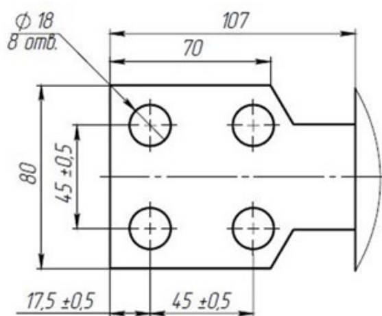
Рис. А.16 – Общий вид трансформатора тока ТПОЛ-СВЭЛ-10М на номинальные первичные токи 2500-3000 А. Остальное см. рис. А.11
