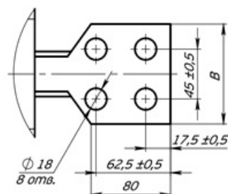
Рис. А.6 – Общий вид трансформатора тока ТПОЛ-СВЭЛ-10 на номинальные первичные токи 2500-3000 А. Остальное см. рис. А.2.
