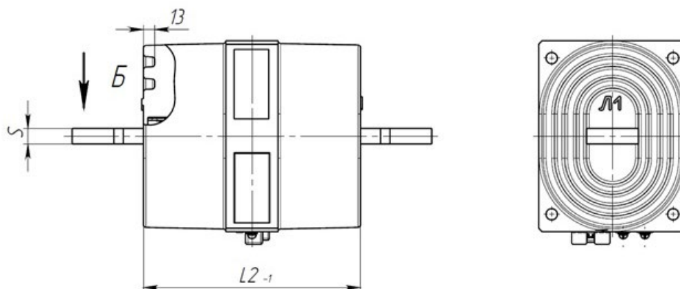
Рис. А.12 – Общий вид трансформатора тока ТПОЛ-СВЭЛ-10М на номинальные первичные токи 1200-2000 А. Остальное см. рис. А.11.
