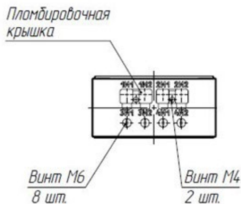
Рис. А.14 – Панель контактов трансформатора тока ТПОЛ-СВЭЛ-10М-4. Остальное см. рис. А.11
