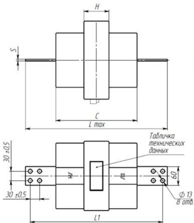
Рис. А.7 – Общий вид трансформатора тока ТПОЛ-СВЭЛ-10-2.1(3.1) на номинальные первичные токи 5-400 А
