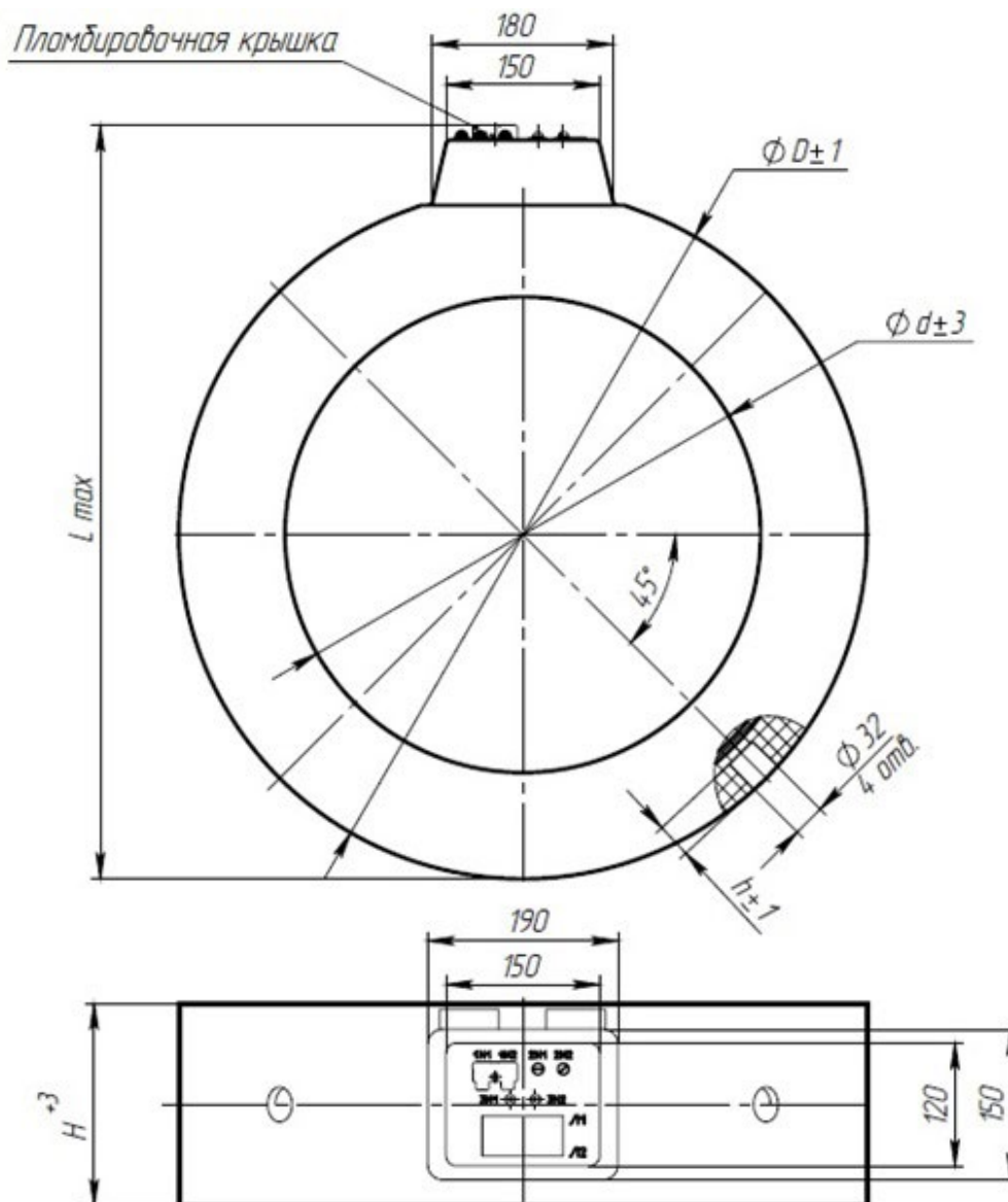
Рис. А.6 – Общий вид трансформаторов ТШЛ-СВЭЛ-10-2.20
