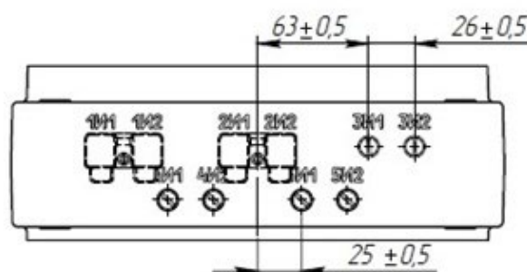
Рис. А.5 – Общий вид трансформаторов ТШЛ-СВЭЛ-10-5. Остальное см. рис. А.1
