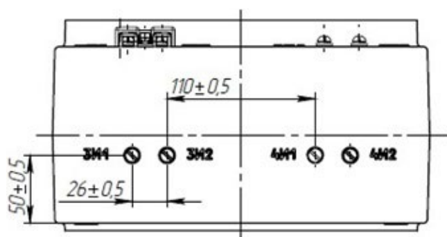
Рис. А.4 – Общий вид трансформаторов ТШЛ-СВЭЛ-10-4. Остальное см. рис. А.1
