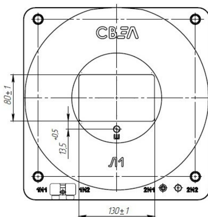
Рис. А.2 – Общий вид трансформаторов ТШЛ-СВЭЛ-10-2.2 Остальное см. рис. А.1.
