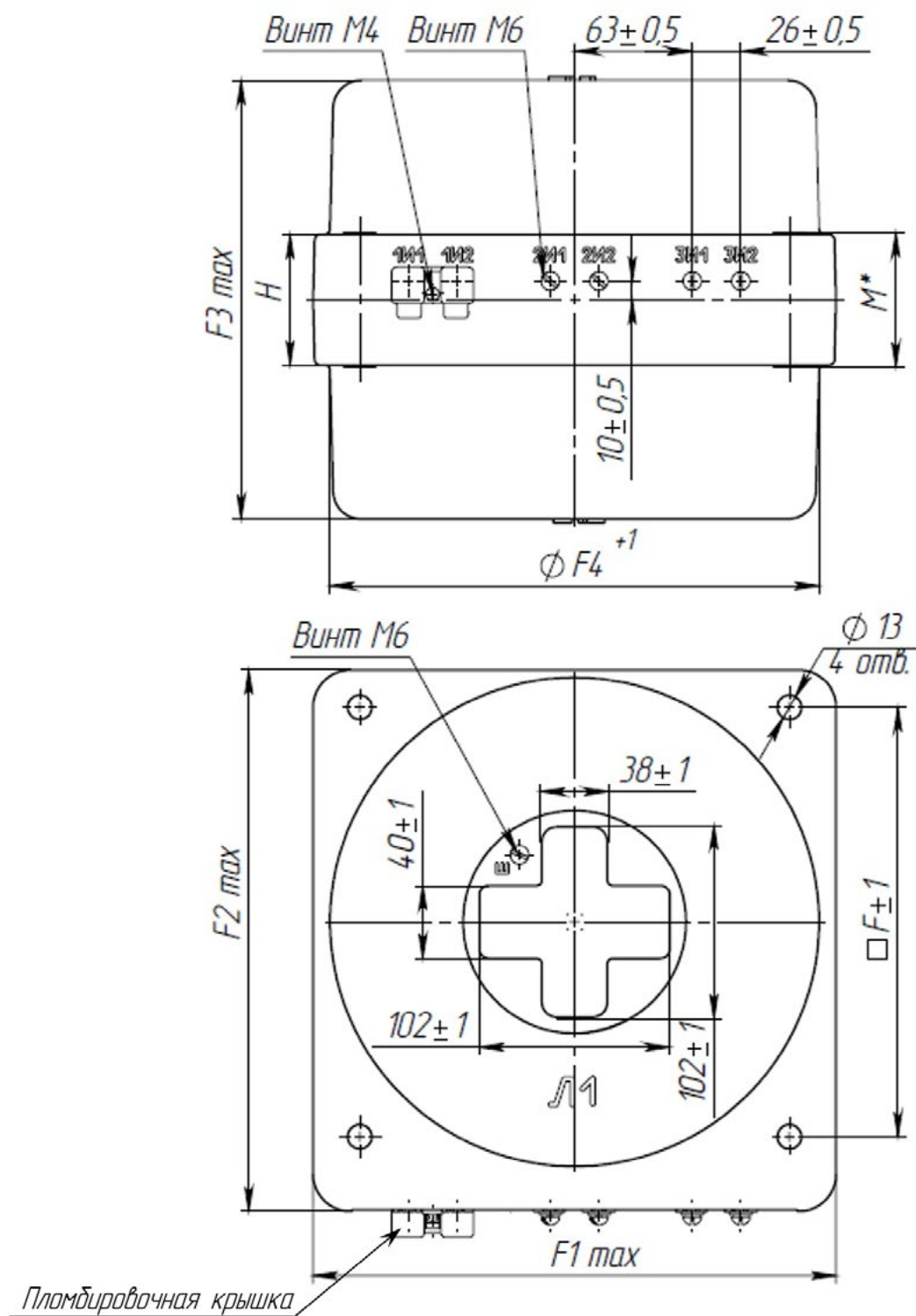
Рис. А.1 – Общий вид трансформаторов ТШЛ-СВЭЛ-10-2.1 и ТШЛ-СВЭЛ-10-3.1
