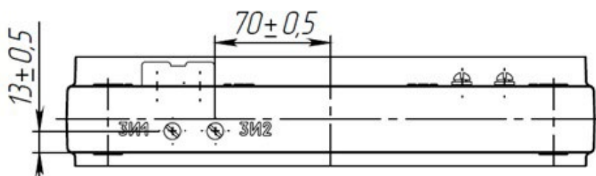
Рис. А.3 – Общий вид трансформаторов ТШЛ-СВЭЛ-10-3.2. Остальное см. рис. А.2
