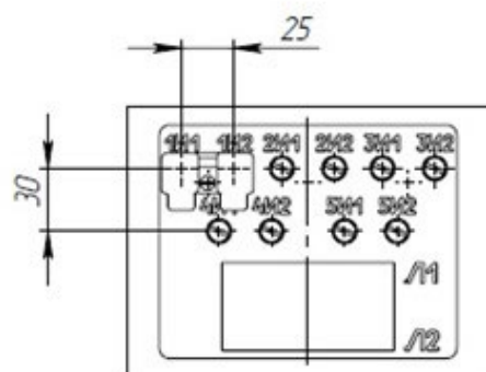
Рис. А.8 – Общий вид трансформаторов ТШЛ-СВЭЛ-20-10-4.20.4.1 (4.20.4.2, 4.20.4.3, 5.20.5.1, 5.20.5.2, 5.20.5.3) Остальное см. рис. А.6
