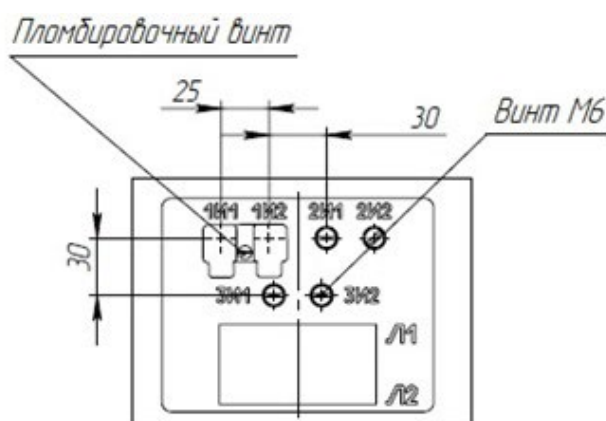
Рис. А.7 – Общий вид трансформаторов ТШЛ-СВЭЛ-10-2.20.2.1 (2.20.2.2, 2.20.2.3, 2.20.3.1, 2.20.3.2, 2.20.3.3) Остальное см. рис. А.6
